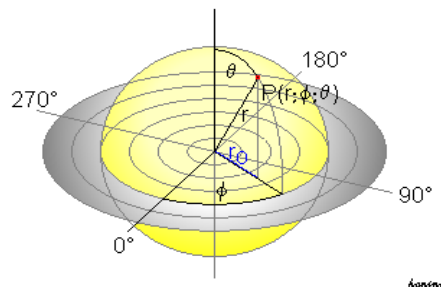
Abbildung 1: Kugelkoordinaten
