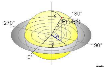
Abbildung 1: Kugelkoordinaten
